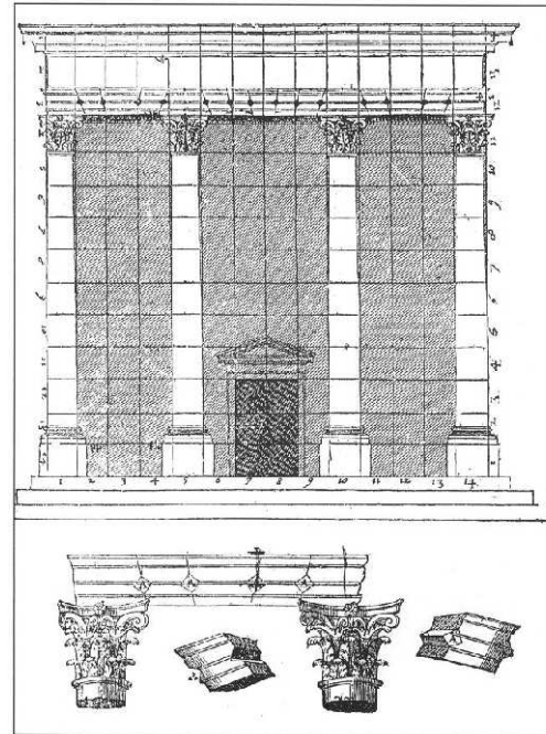
Fig. 16 P. De l'Orme, Architecture . Invenzione di architrave prefabbricata con connettori lapidei.
